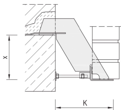
WK-OD mit justierbarer Druckschraube
