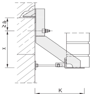
WK-KDS mit grosser DV-Platte
